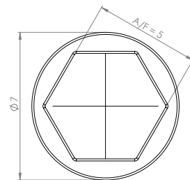
Testa della chiave a bussola
